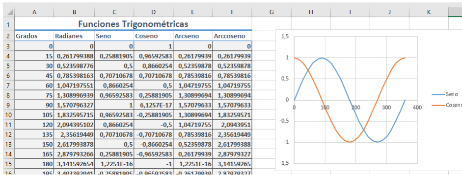
Figura 1: Funciones trigonométricas
